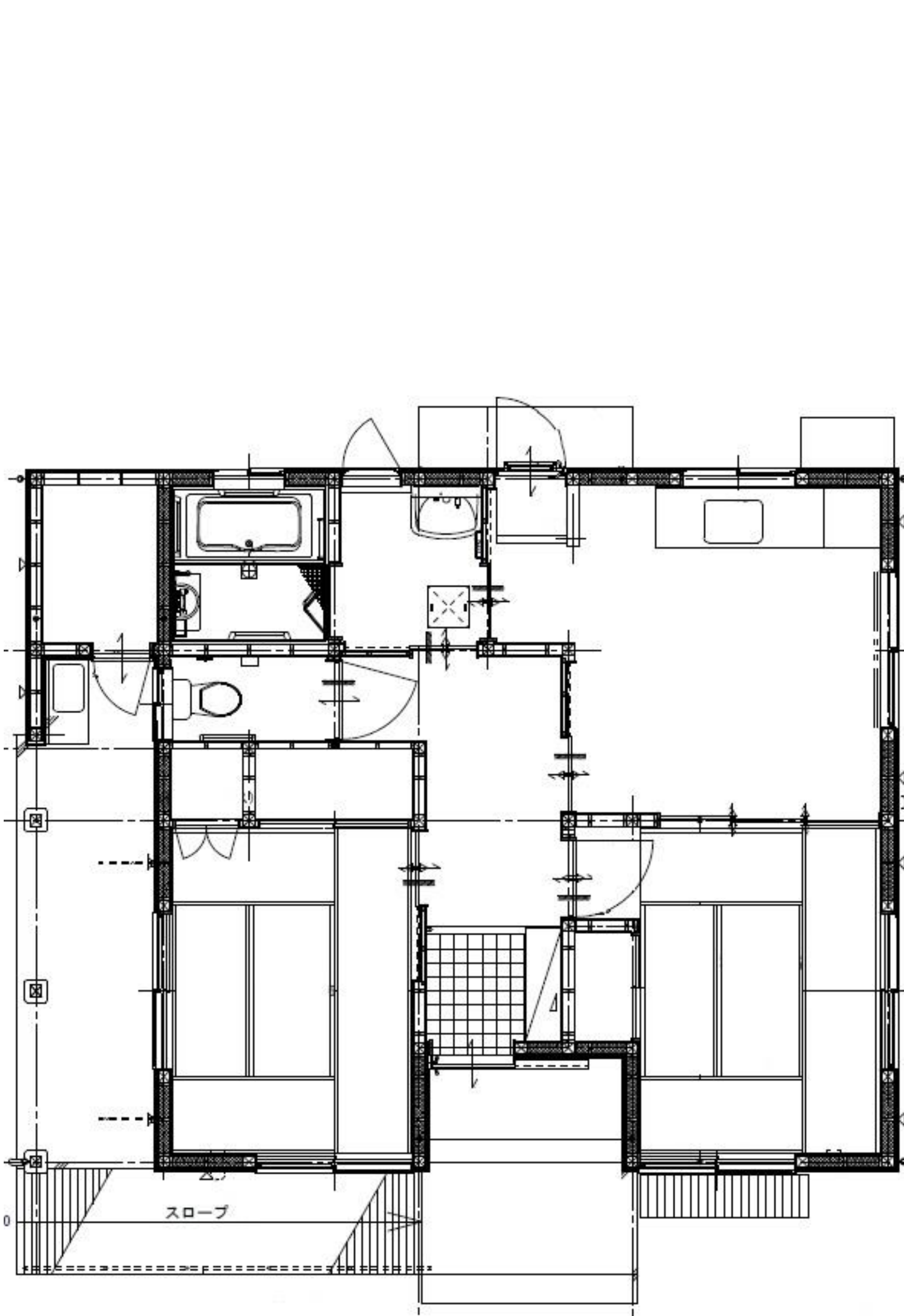
石浜住宅 (2DK)
