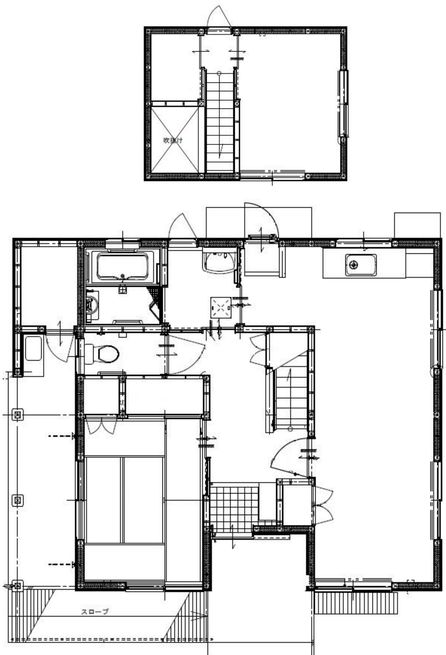
清水住宅 (2LDK)
