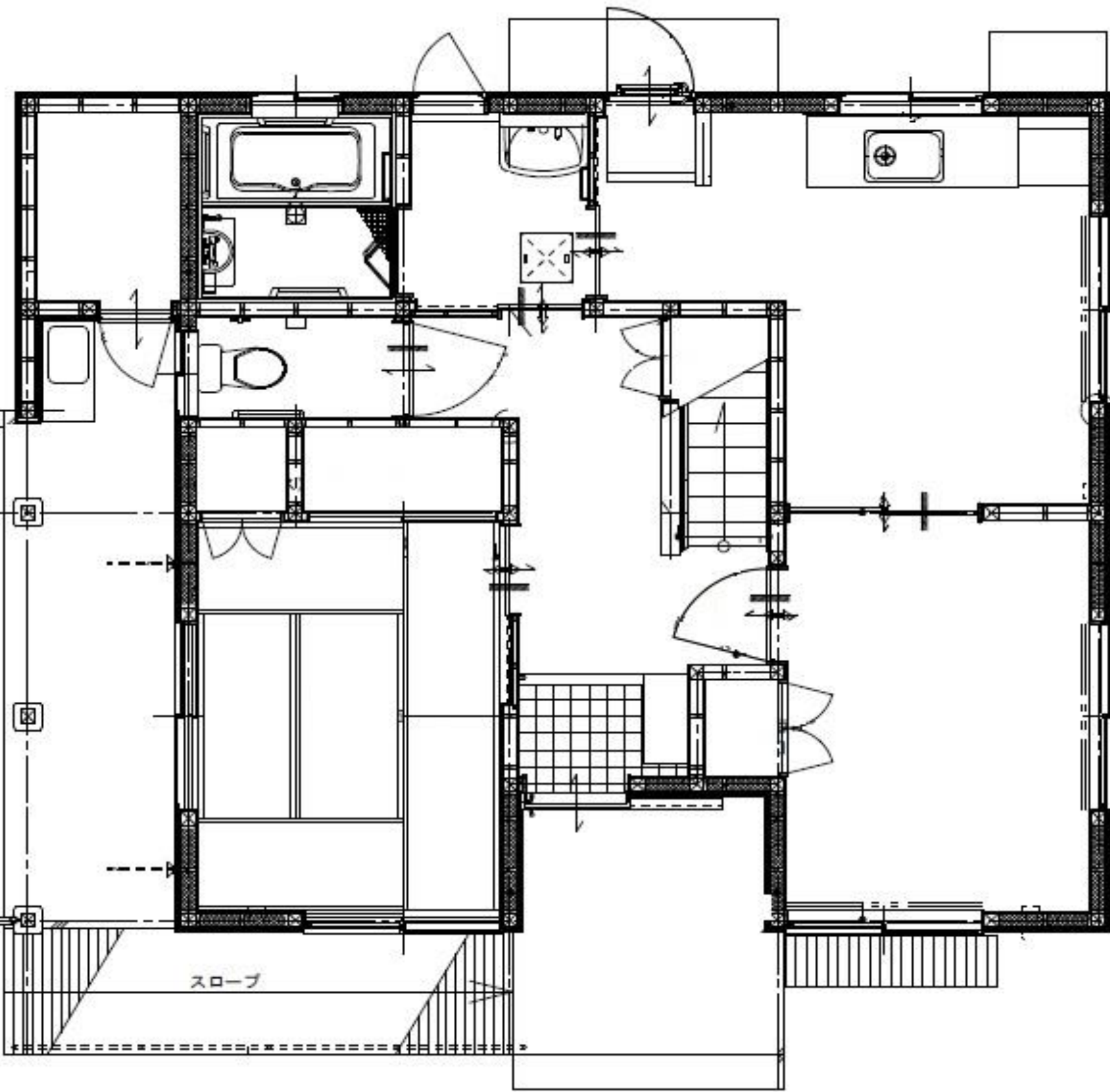
宮ヶ崎住宅 (2DK)
