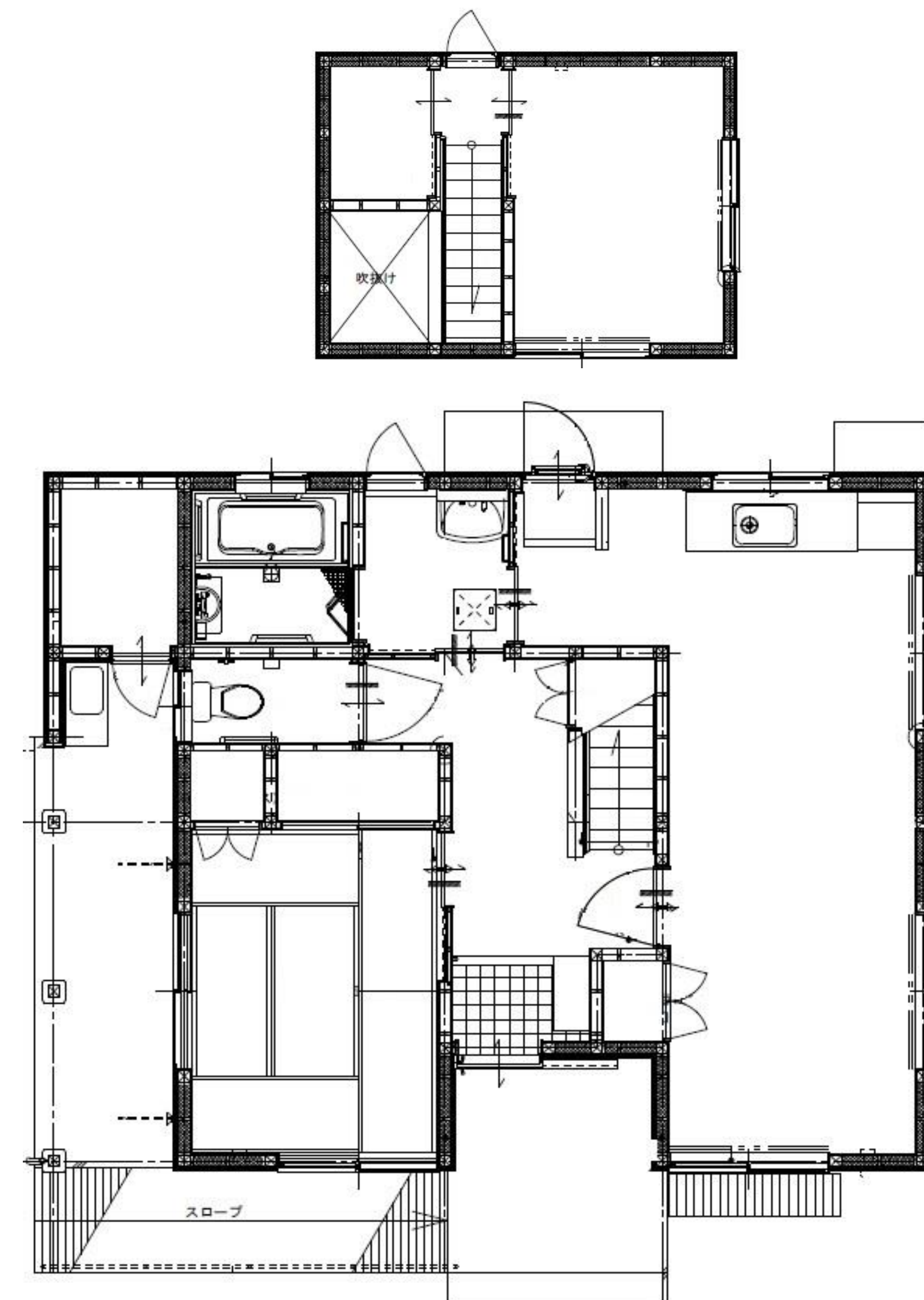
宮ヶ崎住宅 (2LDK)
