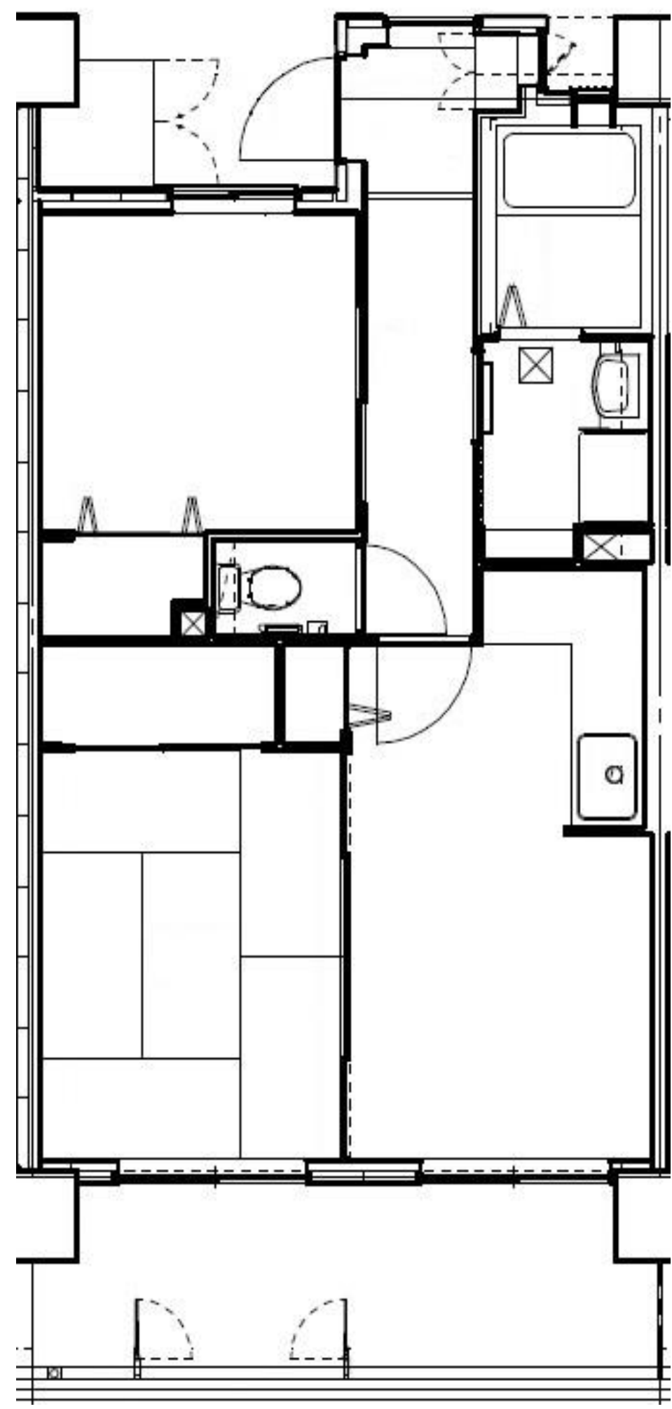
運動公園住宅 (2DK)
