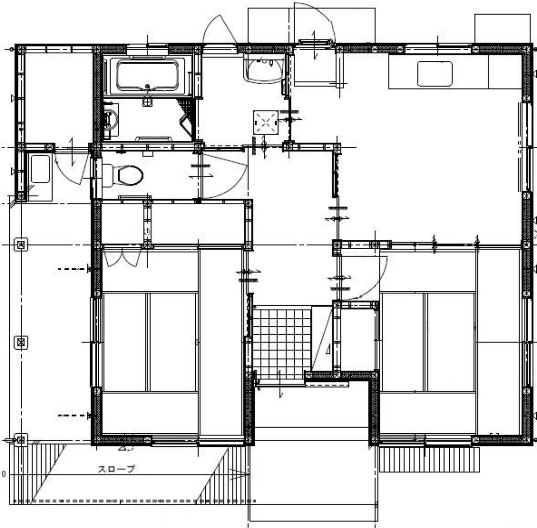
石浜住宅 (2DK)
