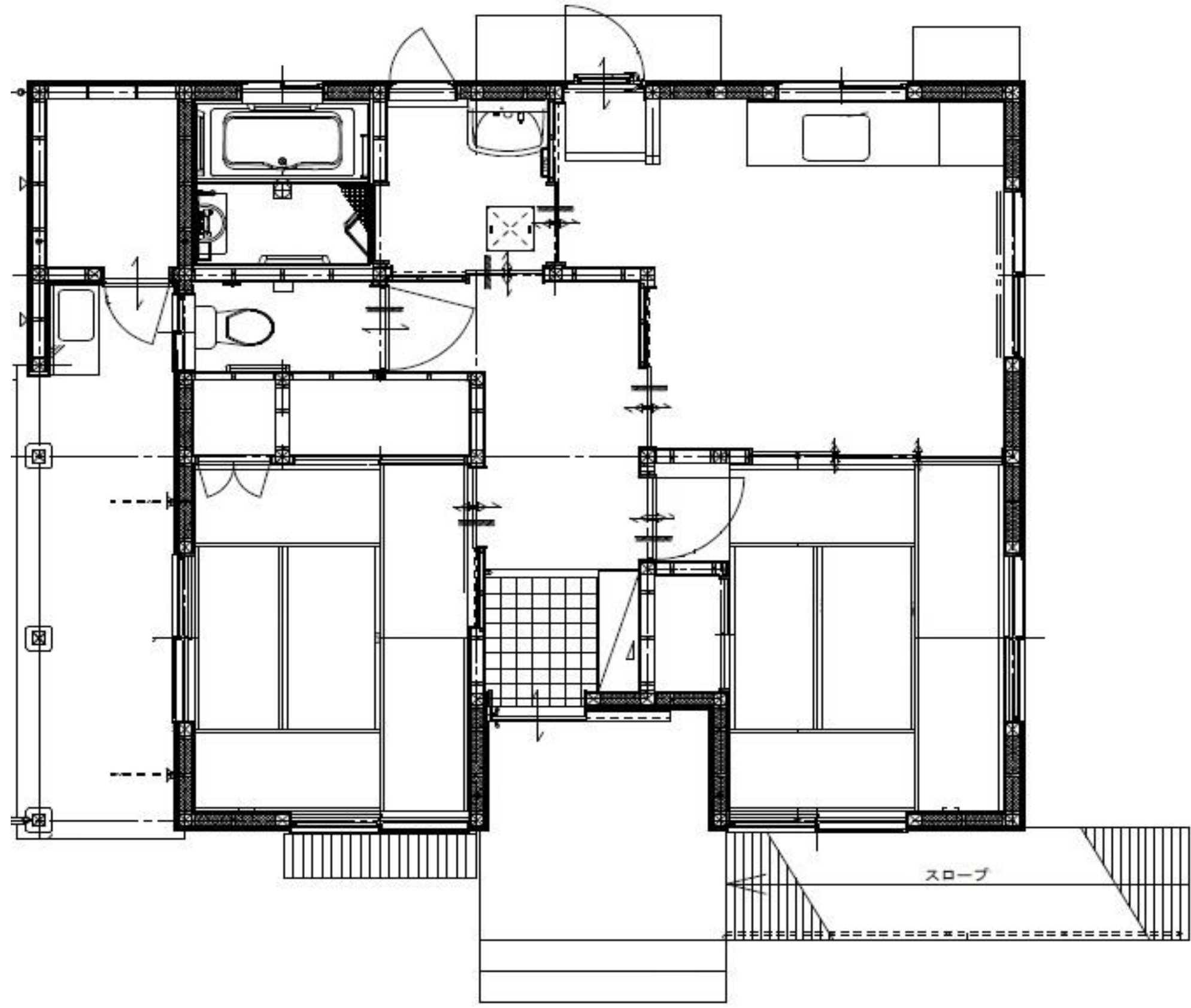
堀切東住宅 (2DK)
