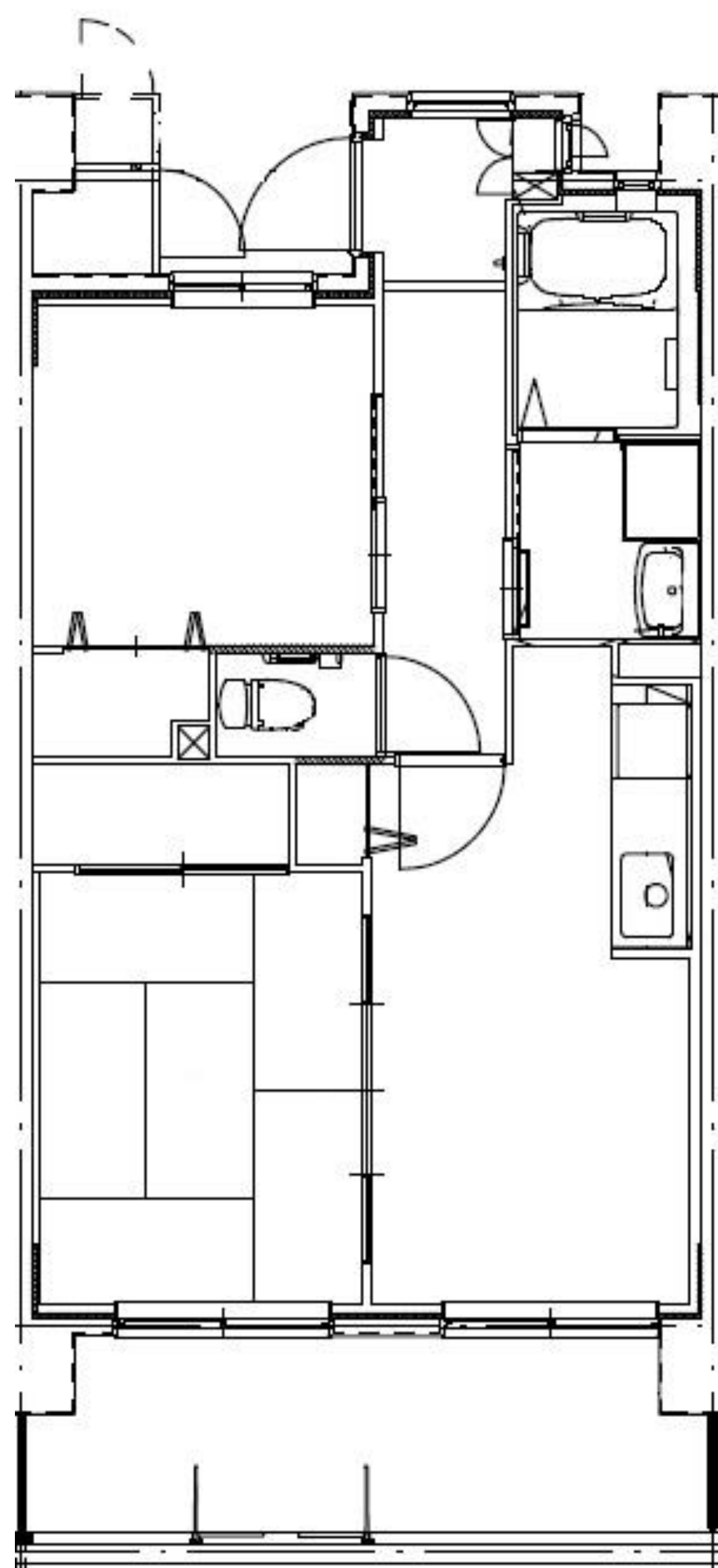
女川住宅 (2DK)
