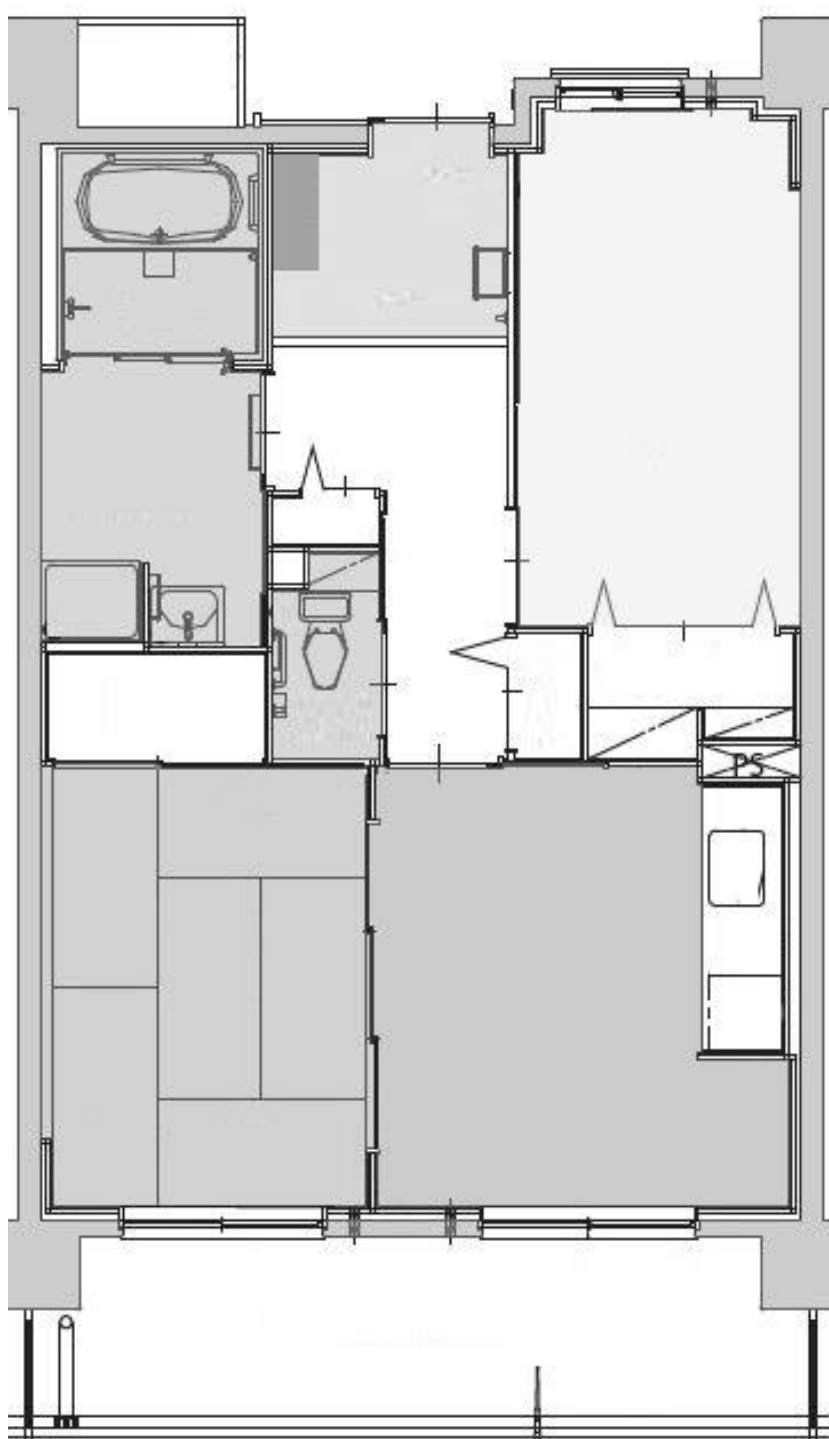
志津川中央復興 2DK
