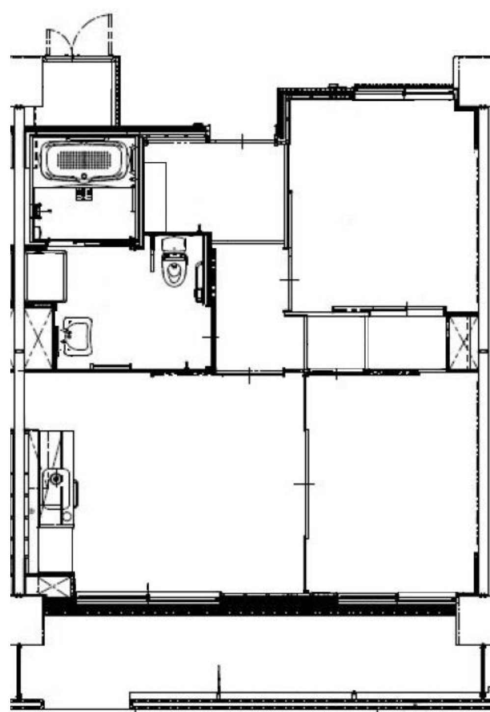
伊里前復興 2DK 車いす
