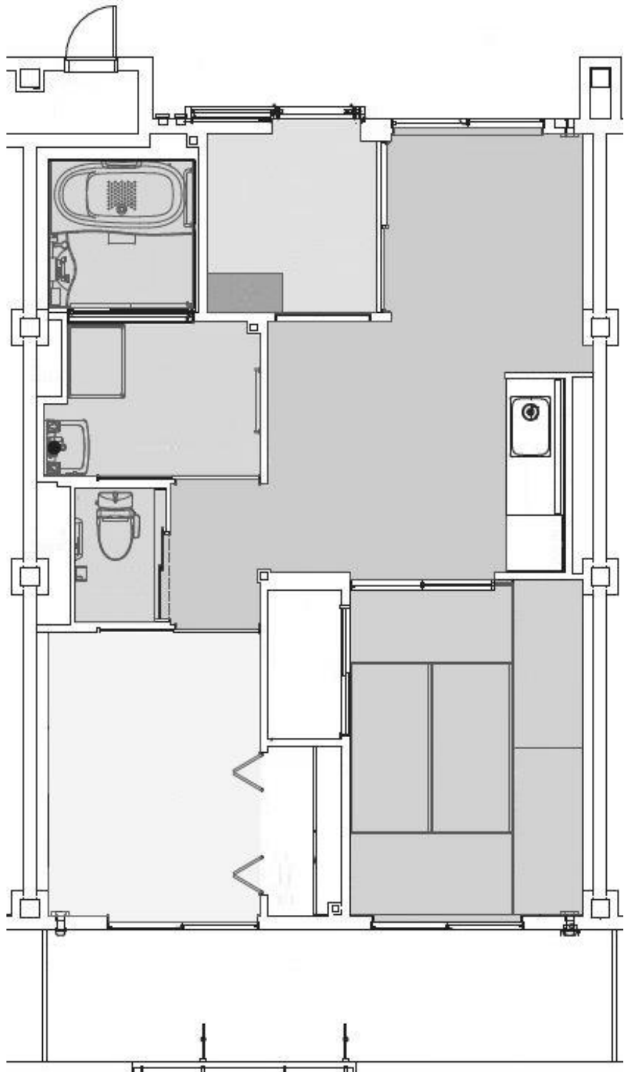
志津川東復興①-B 2DK
