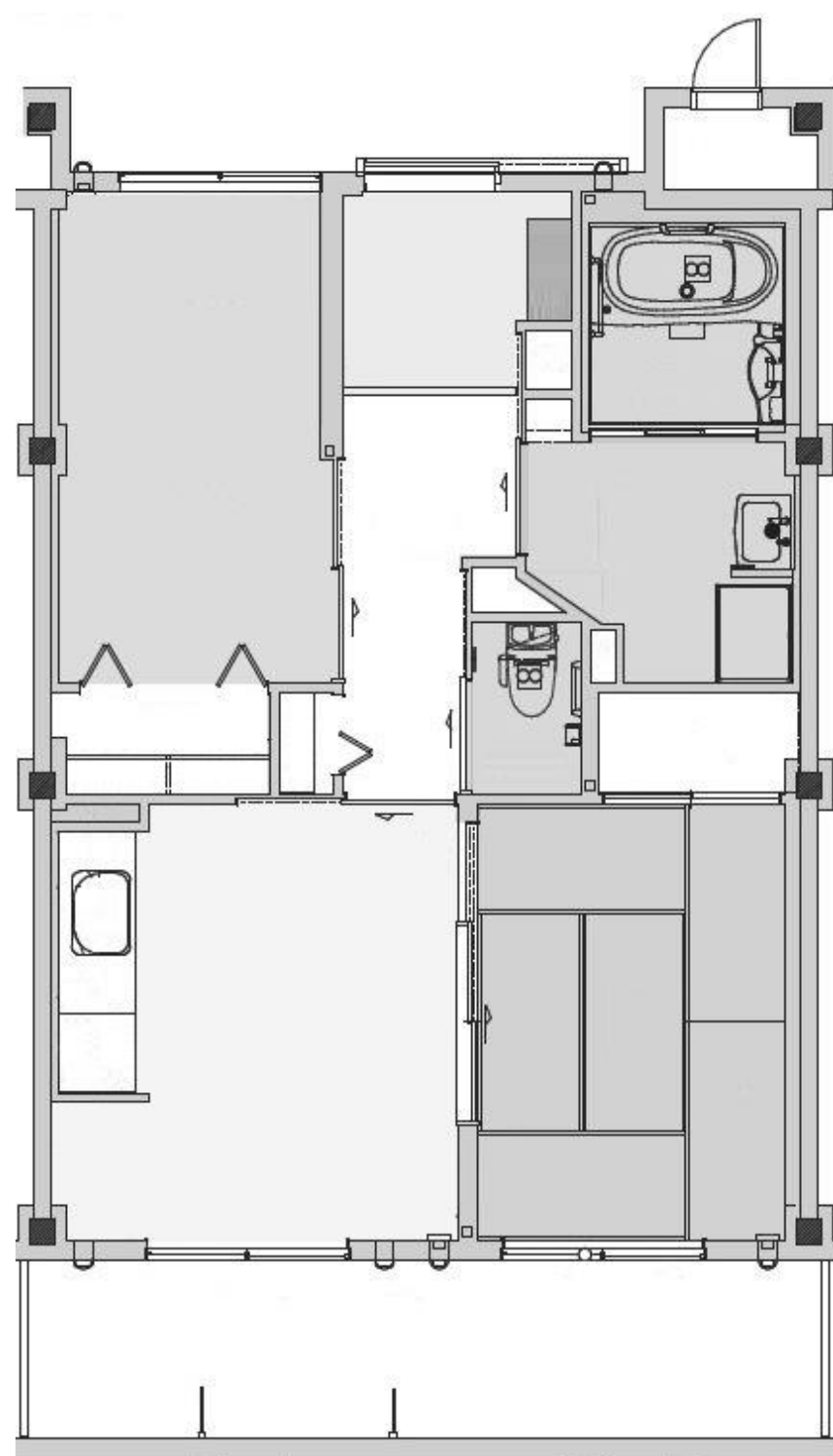
志津川東復興①-A 2DK
