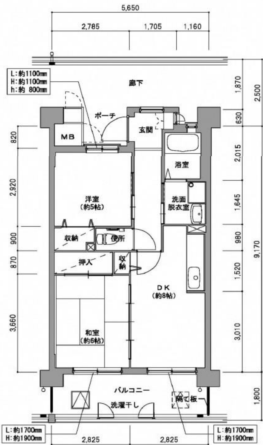
女川住宅 (2DK)
