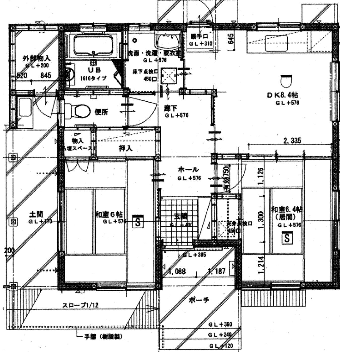
清水住宅 (2DK)
