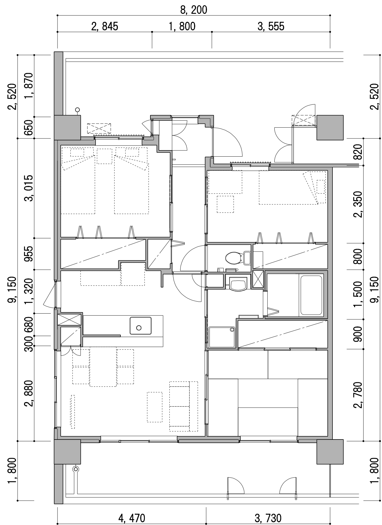
運動公園住宅 (3LDK)
