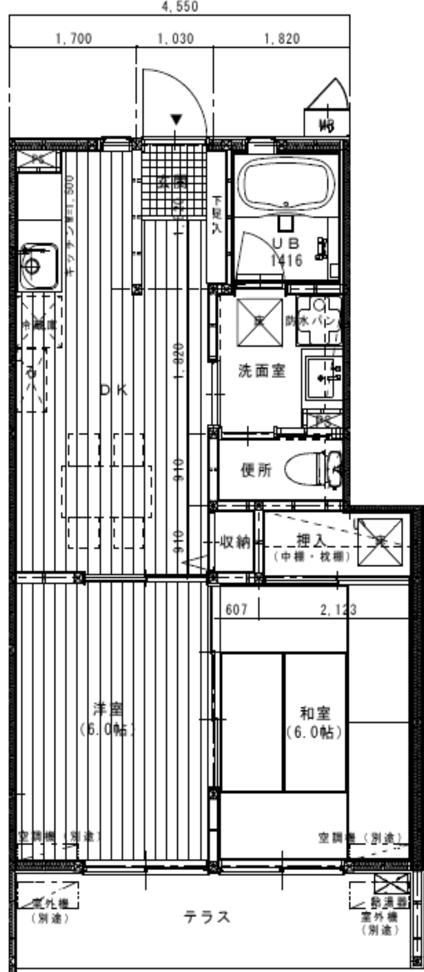
浦宿第二住宅 (2DK)
