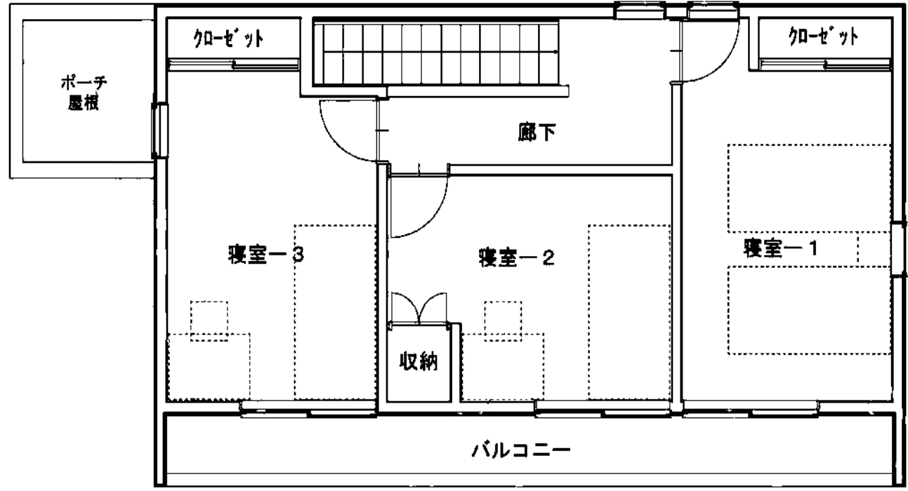
2階
