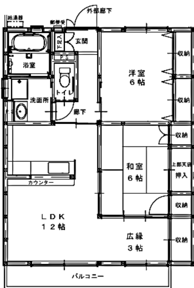
(長屋65㎡タイプ) 面瀬中央②、③
