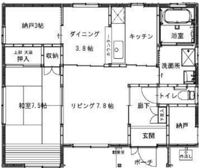
(戸建55㎡タイプ) 長磯浜北①・②、津谷街 (1LDK)
